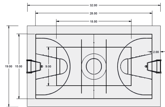
Figura n.º 3. Esquema de losa multiuso tipo I
